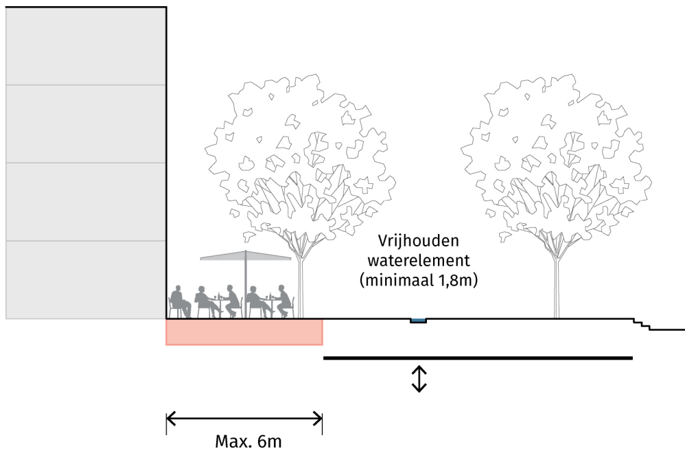
PROFIEL B-B''
