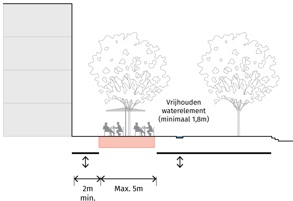
PROFIEL B-B''
